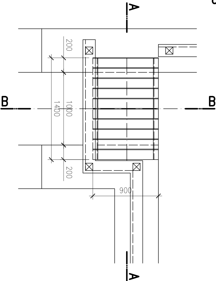
PŮDORYS
